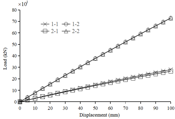
Fig. 17. Displacement-load
