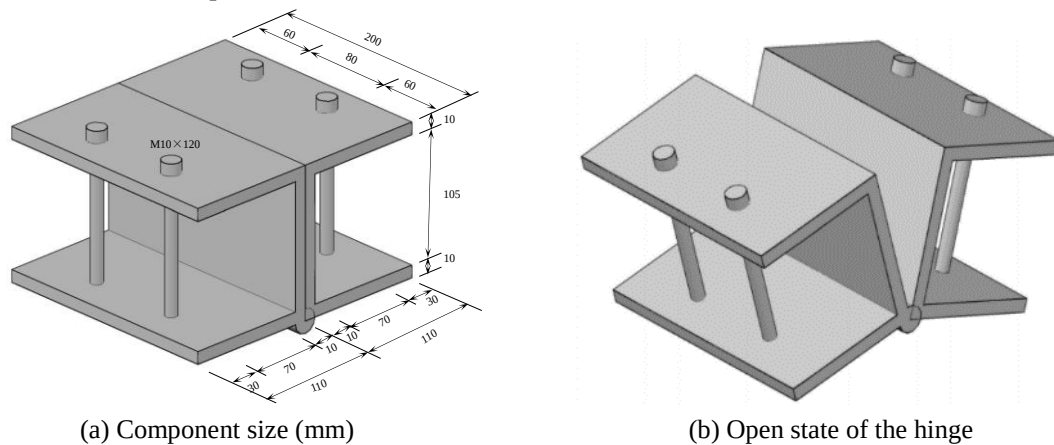
Fig. 20. Steel component
